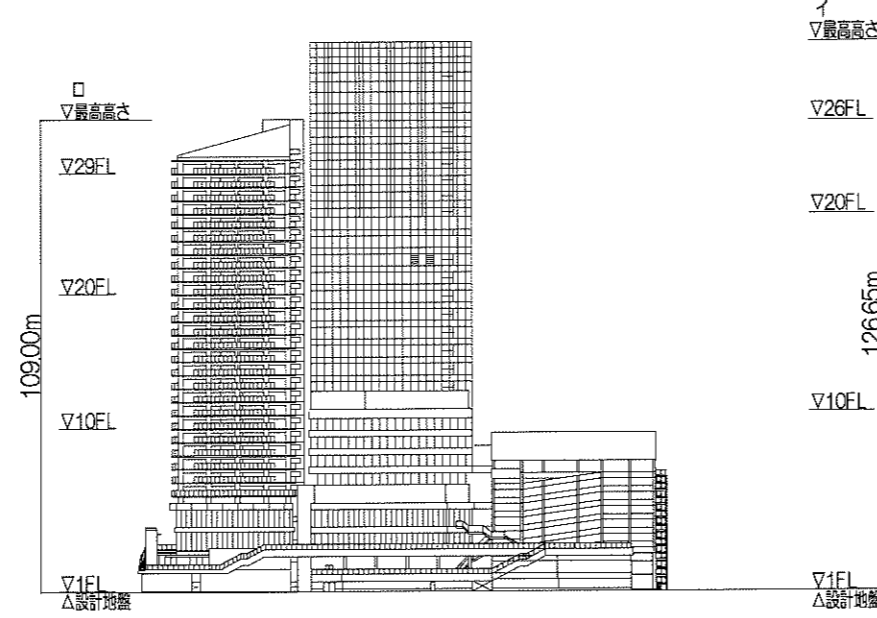
断面位置 (NO SCALE)
