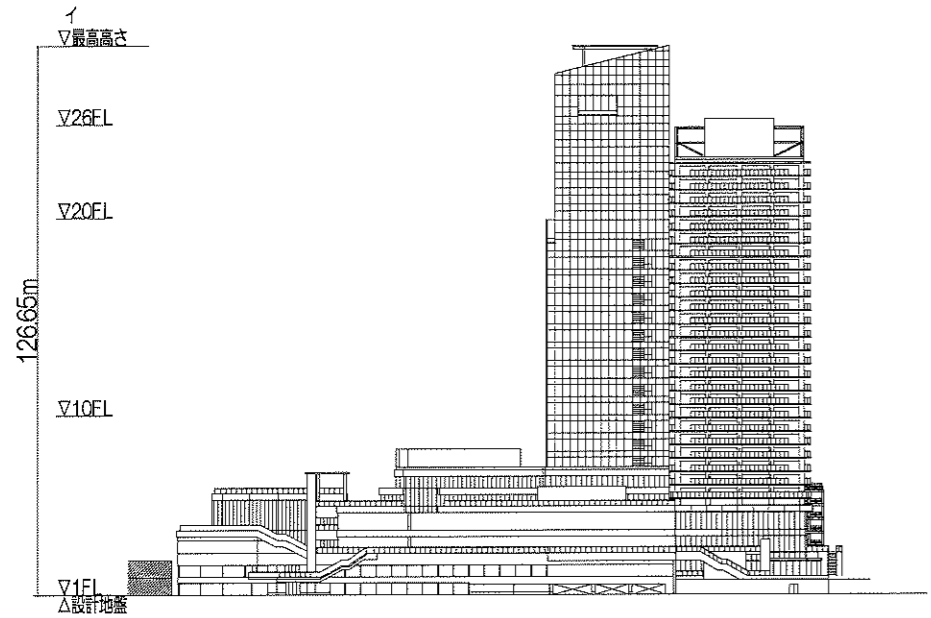
立面方向 (NO SCALE)
